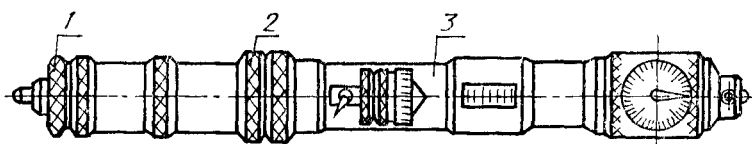
1—измерительный наконечник; 2—удлинитель; 3—микрометрическая головка с индикатором
